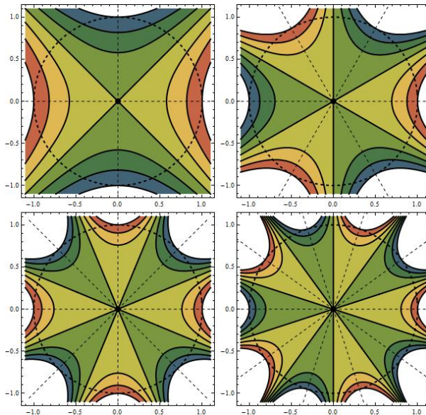
FIGURE 6. Courbes de niveau des fonctions f_{2,1} à f_{2,4} autour de l'origine
